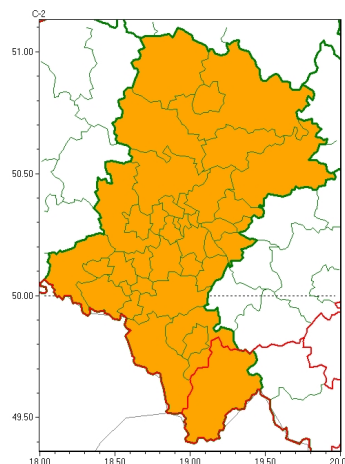
Upał 2026-08-03 05:52
