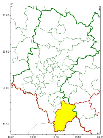
Burze 2026-08-03 05:52
